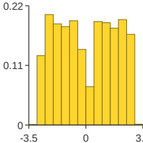
DoS
