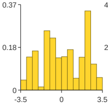
DoS
