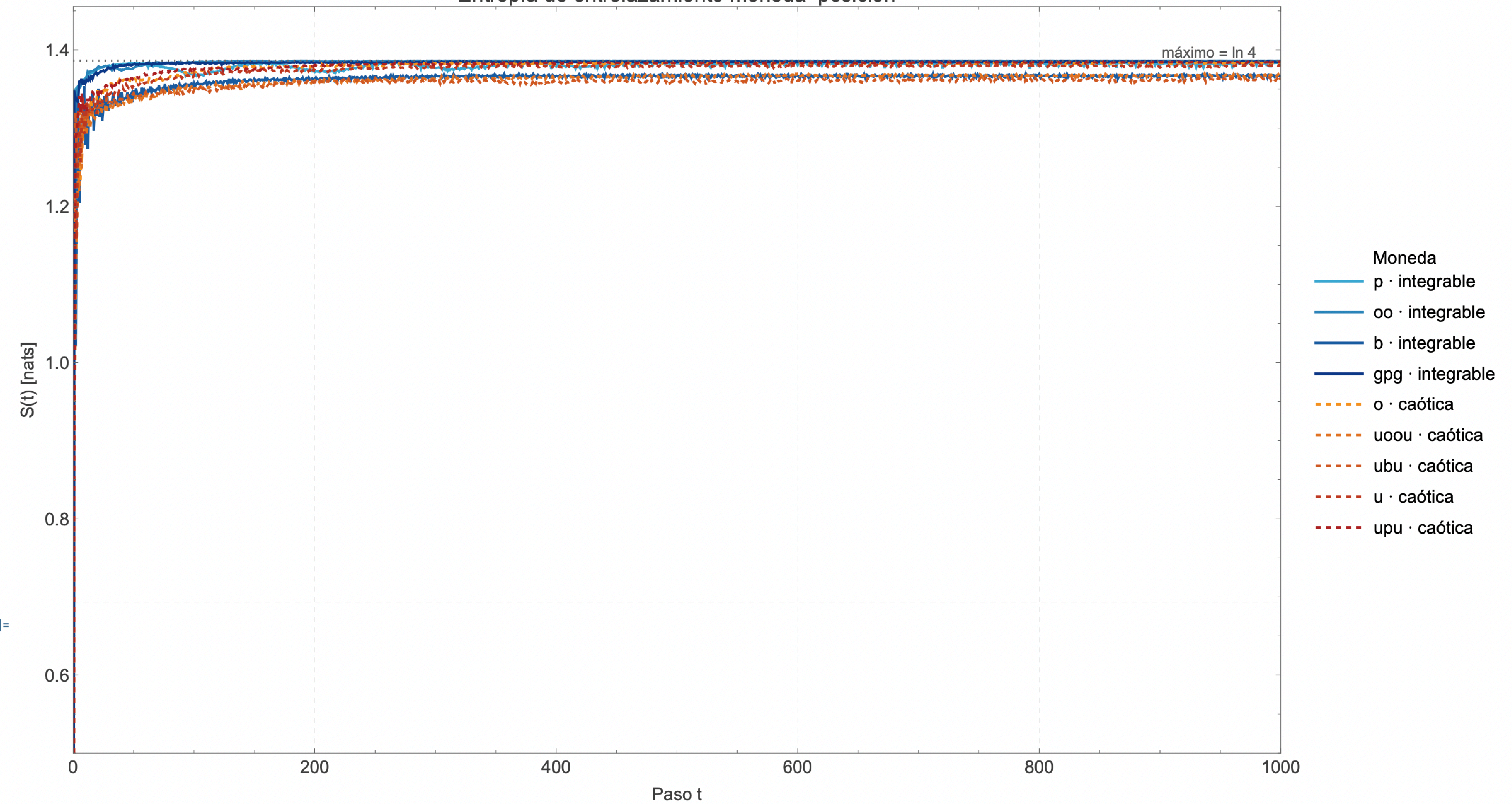
Entropía de entrelazamiento moneda–posición
