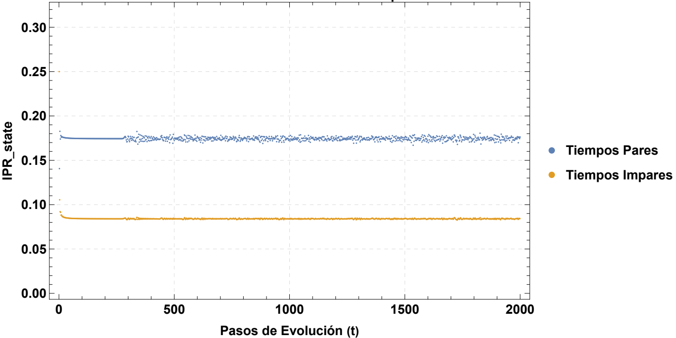
IPR Bunimovich: Bifurcación Par/Impar
