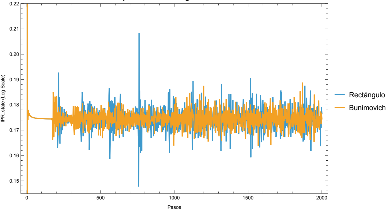
IPR Comparación: Rectángulo vs Bunimovich
