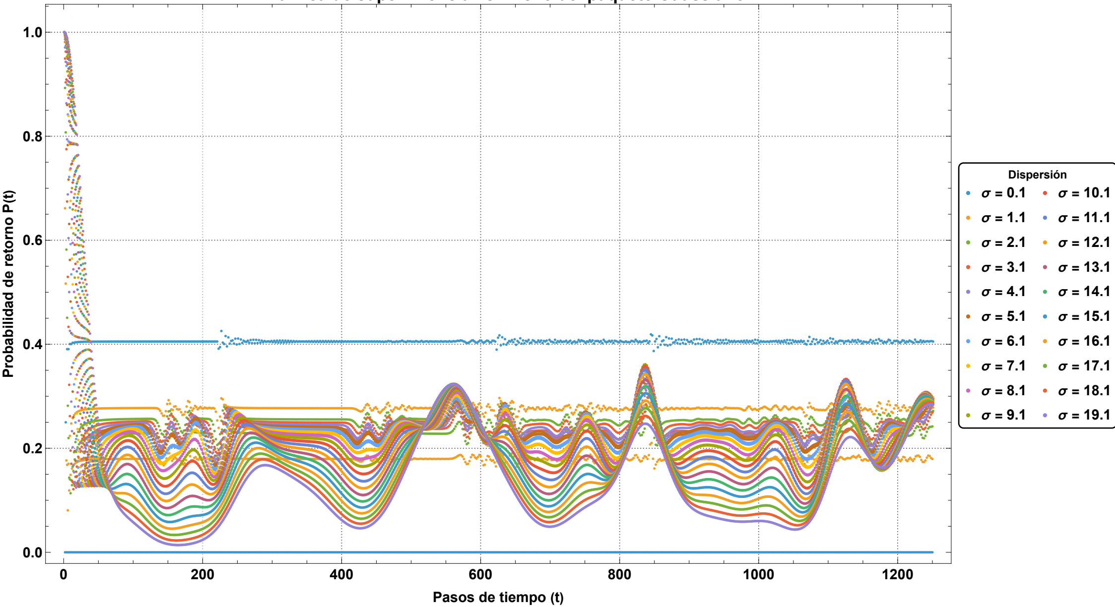
Dinámica de supervivencia vs Ancho del paquete Gaussiano
