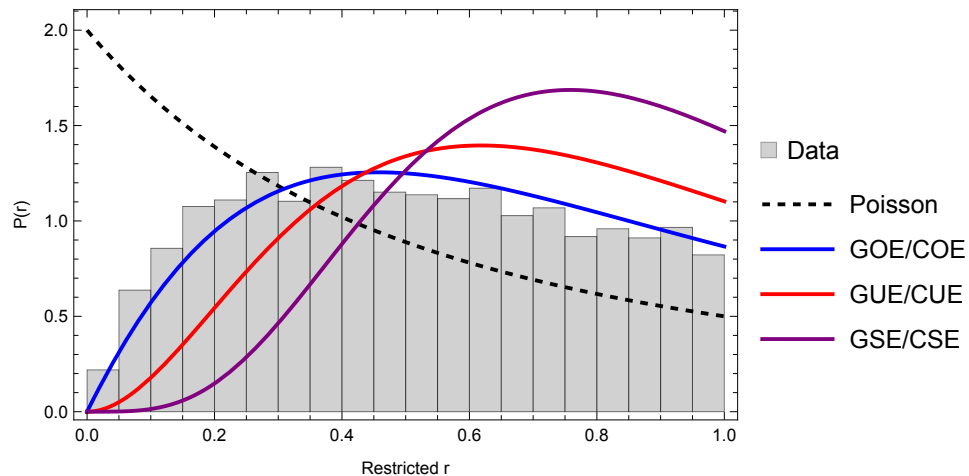
Cocientes de espaciamientos
