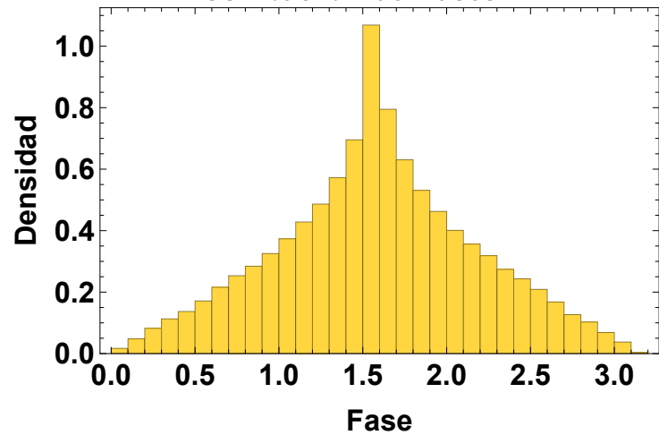
Distribución de fases
