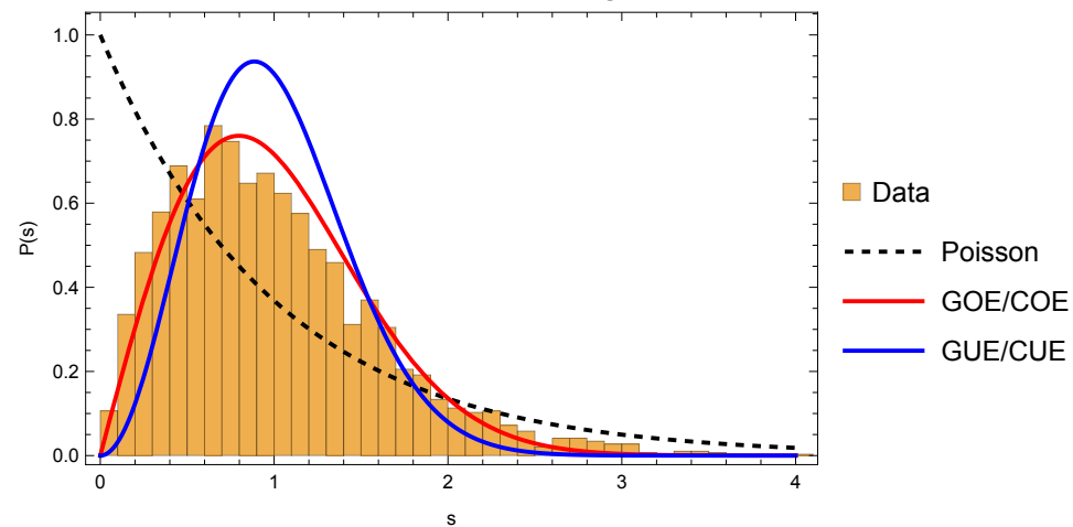
Distribución de espaciamientos
