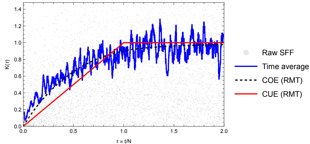
Factor de forma espectral
