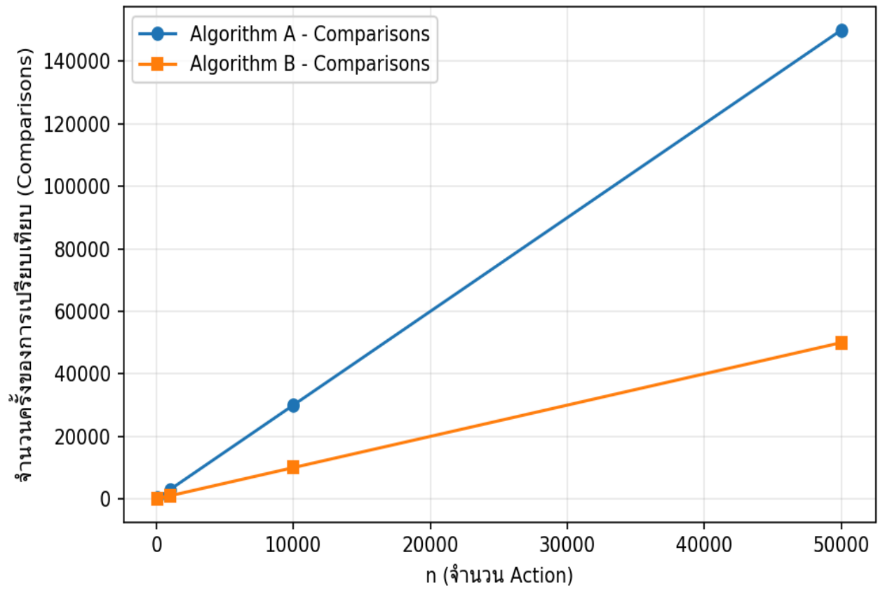
เปรียบเทียบจำนวน Operation (Comparisons) ระหว่าง Algorithm A และ B
