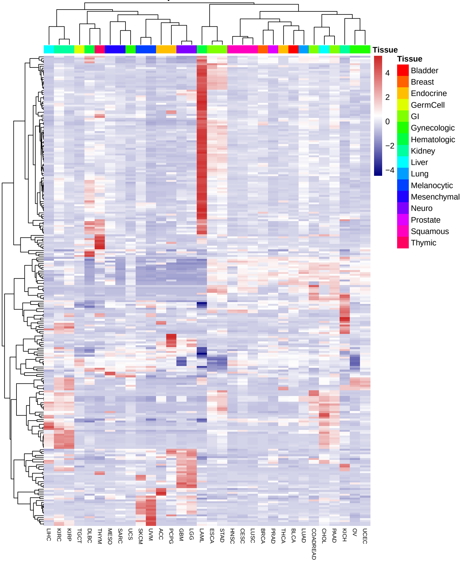
Top 250 Variable SEs
