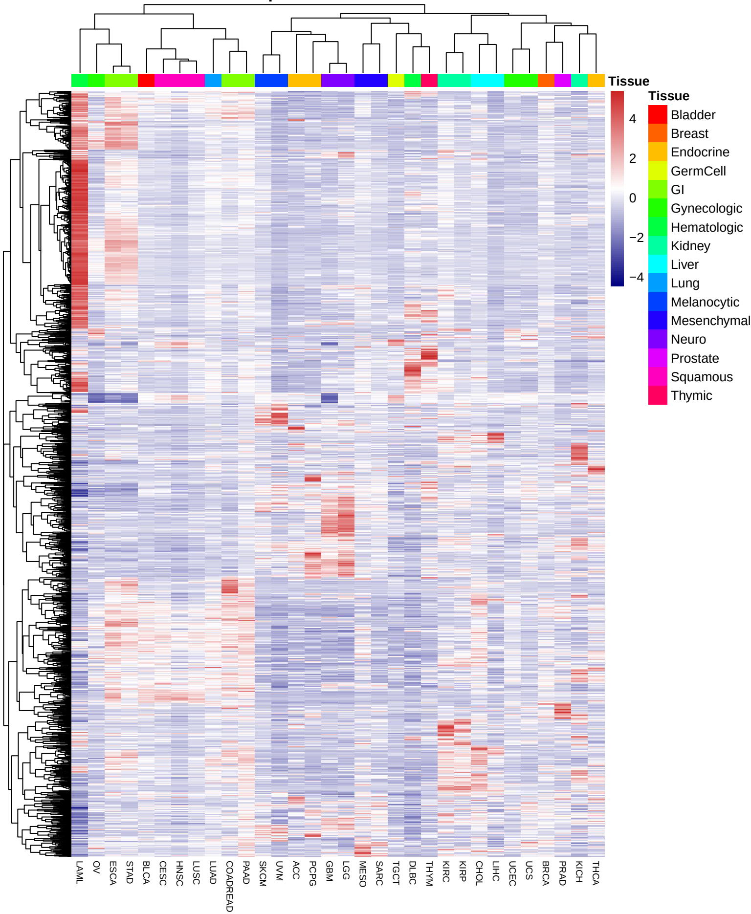
Top 2500 Variable SEs
