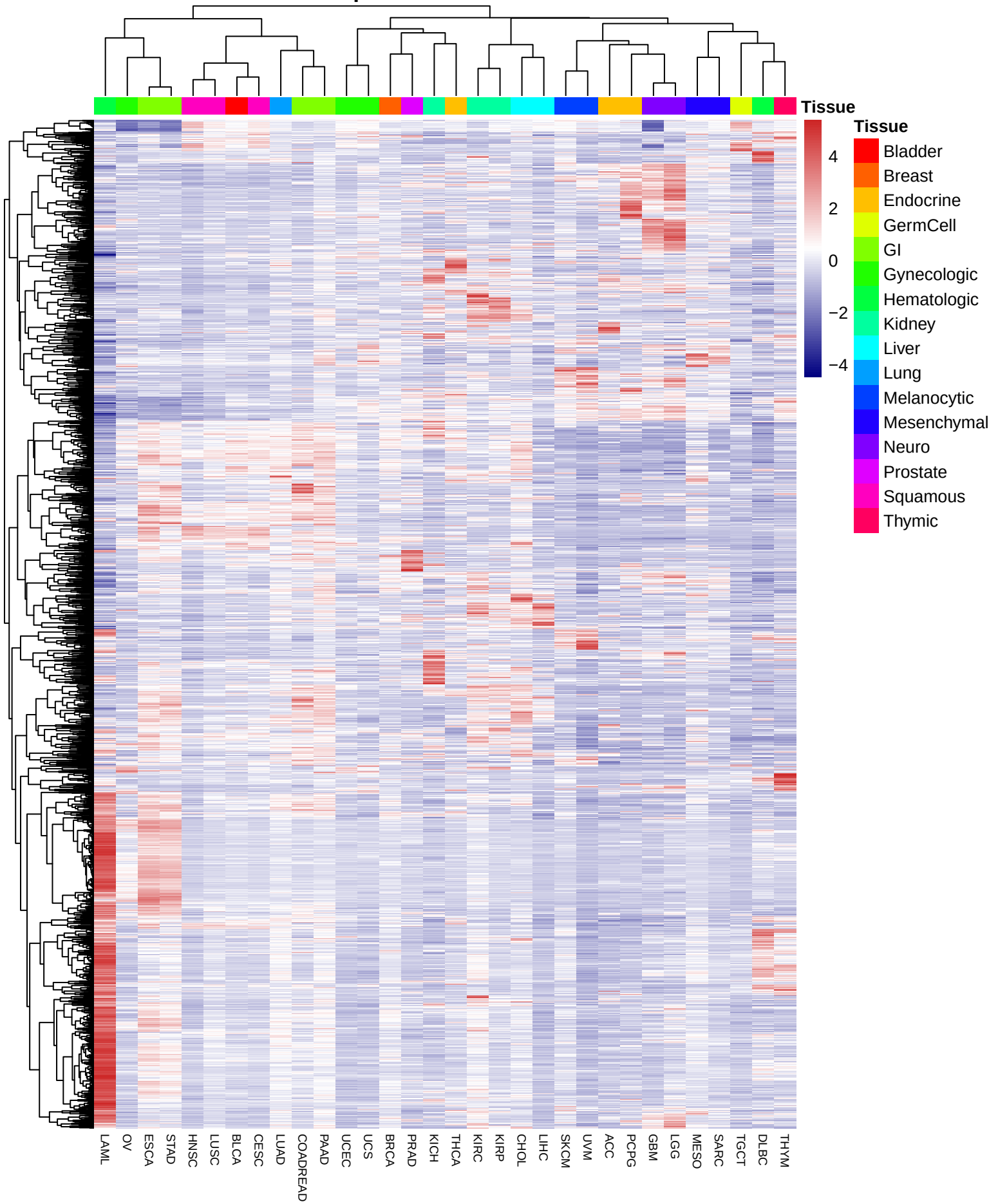
Top 3000 Variable SEs
