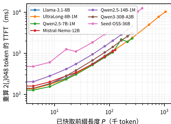
Figure 7: 重算 2,048 個 token 的成本隨已快取前綴長度 P 成長（雙對數軸）。七個模型、每點取 3 次量測的最小值。UltraLong-8B-1M 掃至 1M token。來源： results/m2_harness_mi300x/recompute_position_*.csv 。
