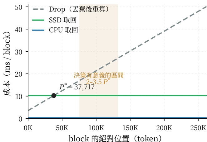
Figure 4: 三個動作的成本結構 (qwen-awq、NVMe)。Cpu 與 Ssd 的取回成本與 block 位置無關，Drop 則線性成長，二者於 P^* = 37,717 token 交叉。底色區為 2-3.5 P^* ，即 P^* 落在請求內部、同一請求的不同位置需要不同決策的長度區間 (§6.8)。
