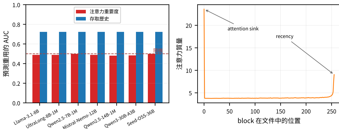
Figure 12: 左：注意力重要度與存取歷史預測「該 block 會被重用」的能力。右：注意力質量隨 block 位置的形狀 (Llama-3.1-8B)。來源：results/m5_attention_mi300x/。
