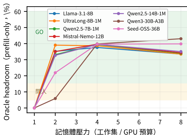
Figure 9: Oracle headroom (prefill-only) 對記憶體壓力。壓力 1x 時為 0% 是正確的退化行為。來源：results/m4_oracle_mi300x/oracle_*.csv。
