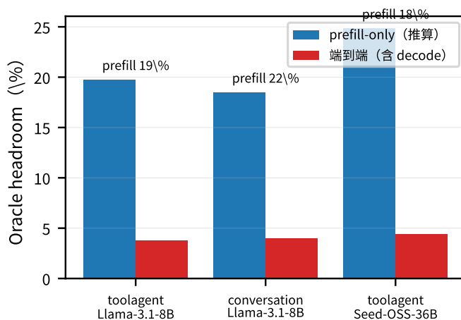
Figure 10: 端到端 headroom 與 prefill-only 的關係。放置決策只能改變 prefill，而 prefill 僅佔總時間的 18–22%。來源：results/m5_predictor_mi300x/policy_sim.csv。
