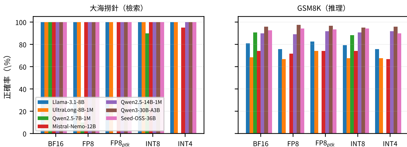
Figure 11: KV 精度的品質代價。左：大海撈針（檢索型）；右：GSM8K（推理型）。同一批精度設定在兩類任務上的 \epsilon 相差兩個數量級。來源：results/m5_quality_mi300x/{needle,gsm8k_precision}_*.csv。
