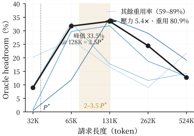
Figure 5: Oracle headroom 隨請求長度的變化 (qwen-awq、NVMe、僅計 prefill)。粗線為固定壓力 (5.4×) 與重用率 (80.9%) 的掃描，細線為其餘三個重用率 (59%–89%) 下的量測。四條線的峰值皆落在 2–3.5 P^* 的底色區內，故峰值位置由成本結構決定而非由重用率決定。
