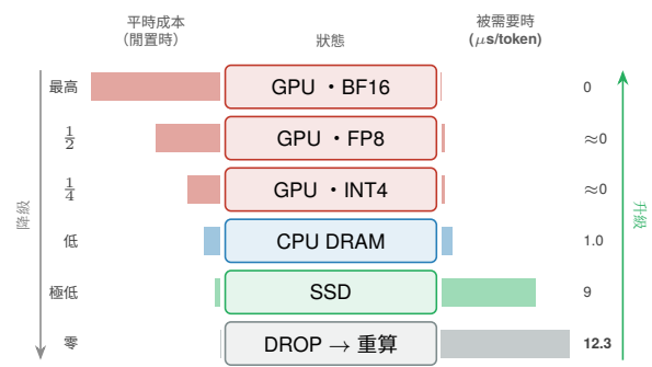
Figure 1: Tiara 的動作空間與其成本結構。與既有工作的差異有二：(i) 位置分層（GPU/CPU/SSD，無損）與精度分層（BF16/FP8/INT4，有損）被統一為單一階梯，而既有工作只做其中之一；(ii) Drop 是階梯上的一層，而非檢索失敗後的補救。兩側長條的長度即為成本，其反向增長是本文的出發點：Drop 閒置時不佔用任何資源，被需要時卻最貴，故其正確性完全取決於未來效用預測。此六階為典型配置之示意，量化器可替換（見第 4 節）。
