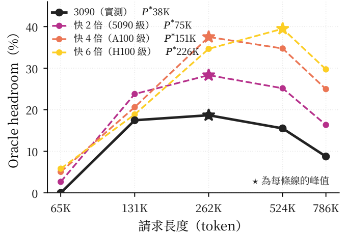
Figure 6: headroom 的峰值隨加速器算力往更長的上下文移動 (壓力 5×、重用率 80.9%、僅計 prefill)。★ 為每條線的峰值：自平台 A 的 262K 移至 6× 算力下的 524K，峰值 headroom 自 18.7% 升至 39.5%。實線為平台 A 的實測；虛線係將實測的 \alpha 按算力倍率縮放，為推算而非量測，其驗證方式見下段。
