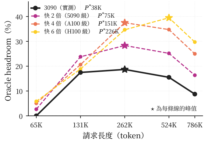
Figure 5: headroom 的峰值隨加速器算力往更長的上下文移動 (壓力 5×、重用率 80.9%、僅計 prefill)。★ 為每條線的峰值：自平台 A 的 262K 移至 6× 算力下的 524K，峰值 headroom 自 18.7% 升至 39.5%。實線為平台 A 的實測；虛線係將實測的 \alpha 按算力倍率縮放，為推算而非量測，其驗證方式見下段。
