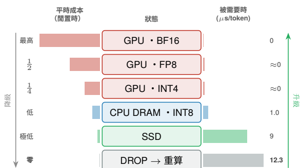
Figure 1: Tiara 的動作空間與其成本結構。與既有工作的差異有二：(i) 位置分層 (GPU/CPU/SSD) 與精度分層 (BF16/FP8/INT4/INT8) 被統一為單一階梯，而既有工作只做其中之一；(ii) Drop 是階梯上的一層，而非檢索失敗後的補救。兩側長條的長度即為成本，其反向增長是本文的出發點：Drop 閒置時不佔用任何資源，被需要時卻最貴，故其正確性完全取決於未來效用預測。此六階為典型配置之示意，量化器可替換 (見第 4 節)。
