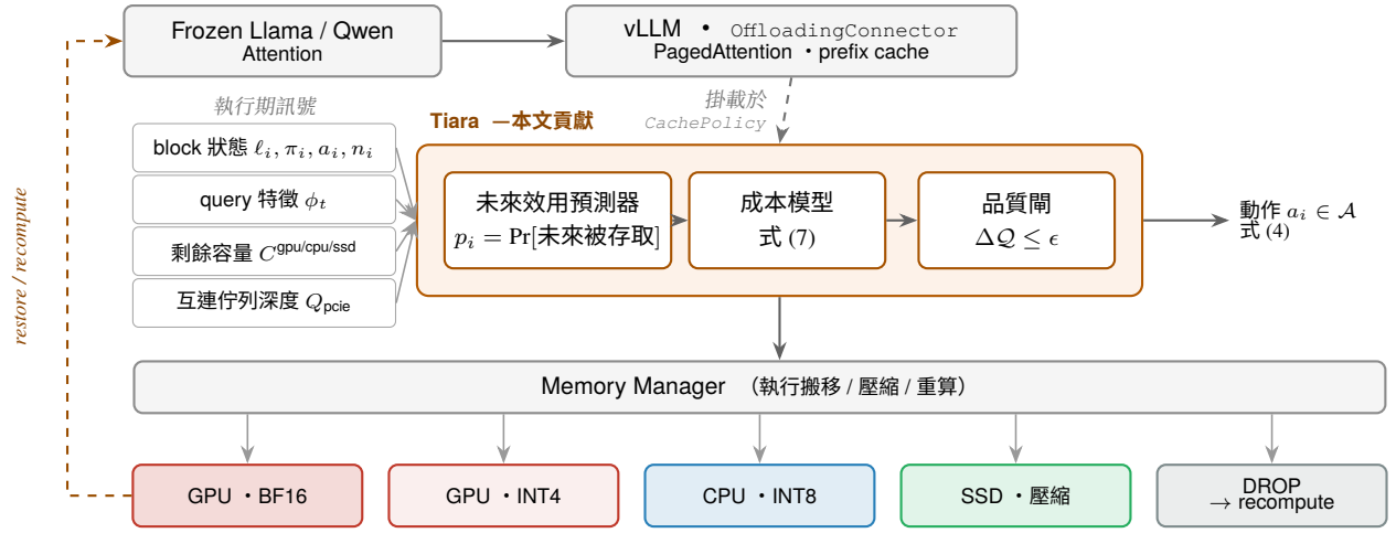
Figure 2: Tiara 架構與資料流。灰底為既有基礎設施，橘框為本文貢獻。控制器接收四類執行期訊號，經「未來效用預測 → 成本模型 → 品質閘」三階段，為每個 KV block 產生一個動作 a_i \in \mathcal{A} ，交由 Memory Manager 執行。關鍵設計決定是不自行實作推論引擎：Tiara 掛載於 vLLM 既有的 CachePolicy 介面，貢獻邊界因而清晰（機制屬於 vLLM，策略屬於本文），且可在 CUDA 與 ROCm 上零移植部署，並直接與內建的 lru/arc 對照。左側橘色虛線為恢復路徑：被降級或丟棄的 block 在重新變得重要時可升回上層或重算，單次誤判不會造成資訊的永久損失。
