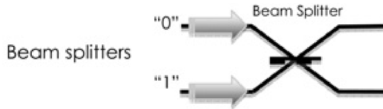
Figure 3: Darstellung einer Dual-Rail Kodierung mit einem 50:50 Strahlteiler[4].
