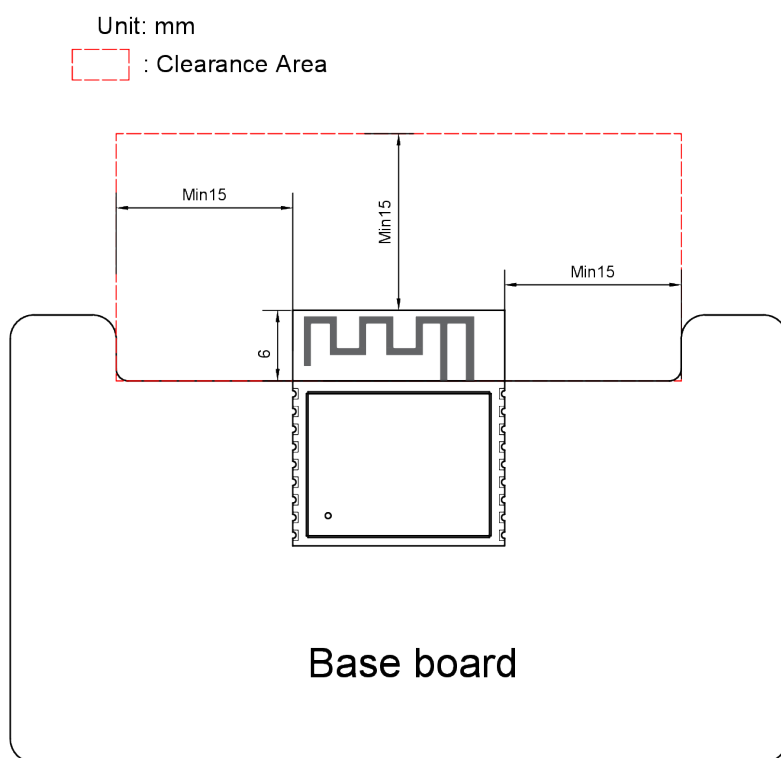
图 21: ESP32-C3 系列模组 (天线馈点在左侧) 天线区域净空示意图
