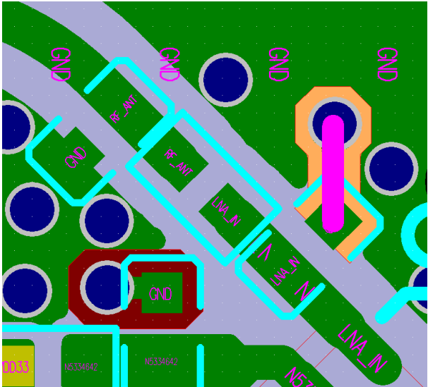
图 16: ESP32-C3 系列芯片四层板射频短截线设计
