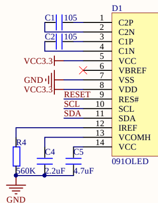
OLED显示控制电路
