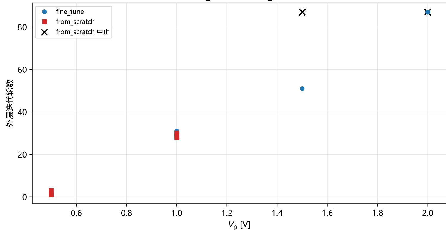
全 SP 循环: fine_tune vs from_scratch 收敛轮数
