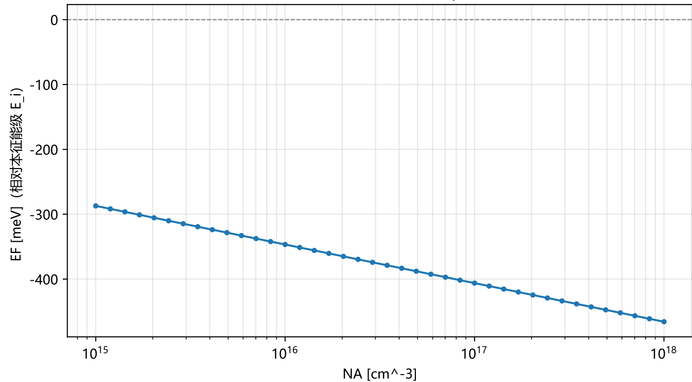
费米能级随掺杂浓度变化 (p 型)
