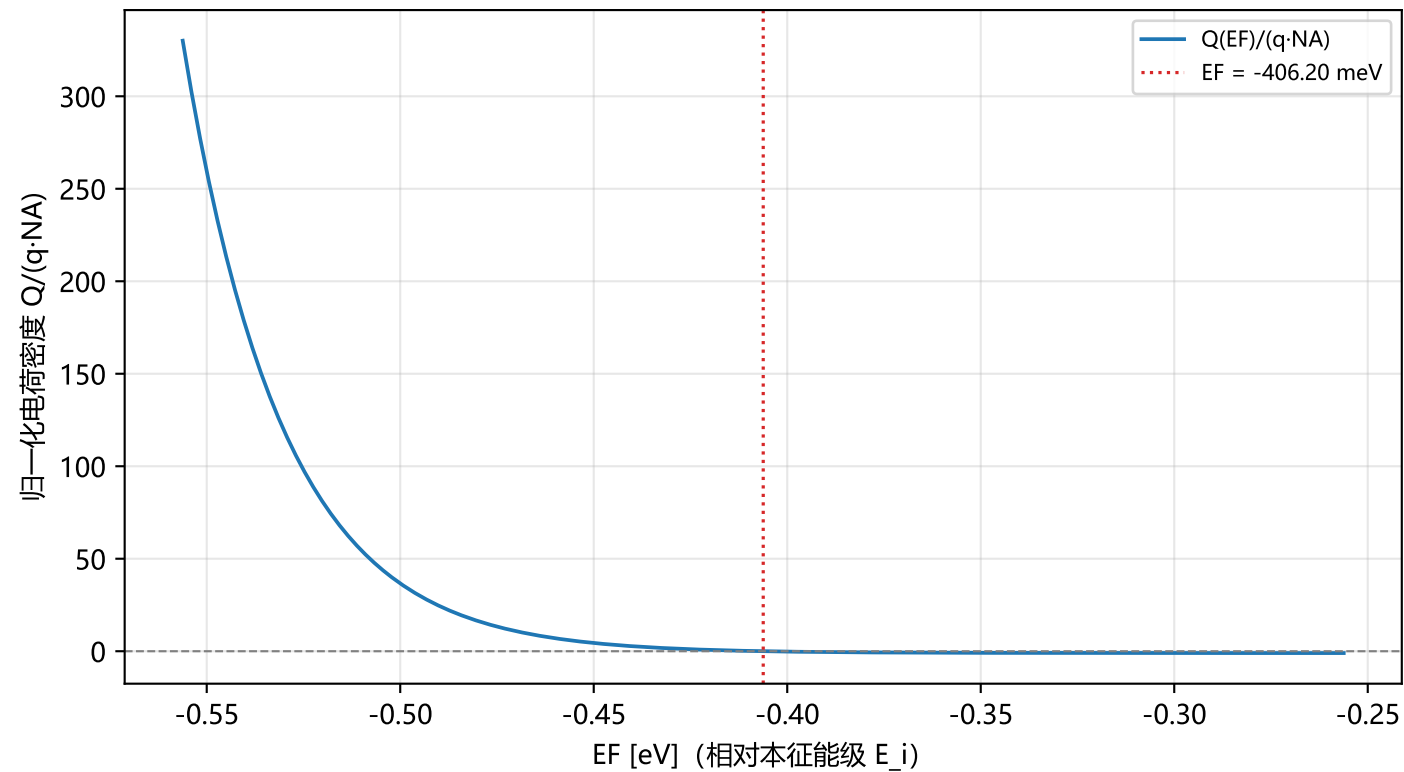
bulk 电中性: Q(E_F) 单调递减、穿越零点
