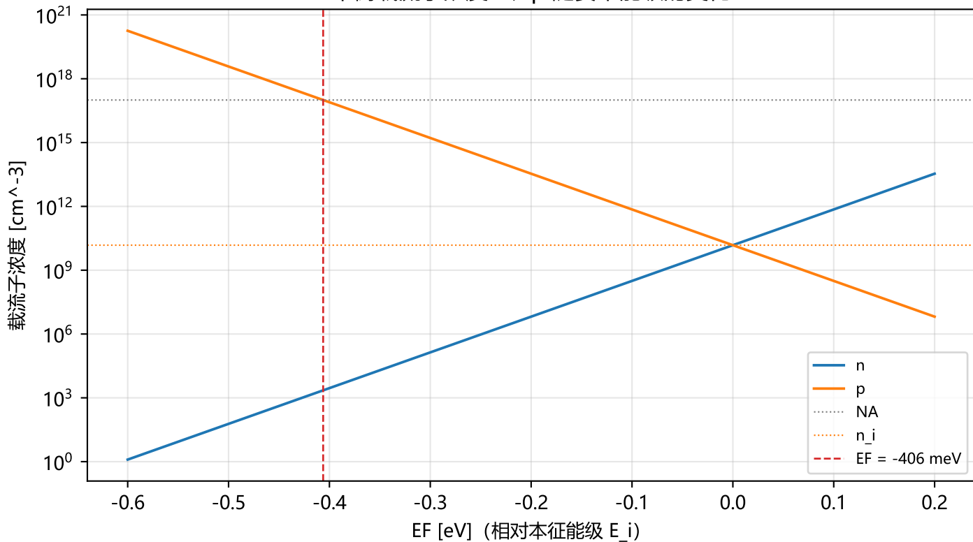
平衡载流子浓度 n 、 p 随费米能级的变化
