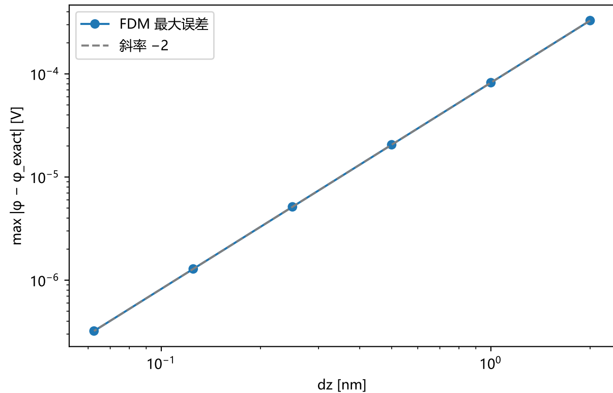
Poisson-FDM 收敛阶 (光滑问题)
