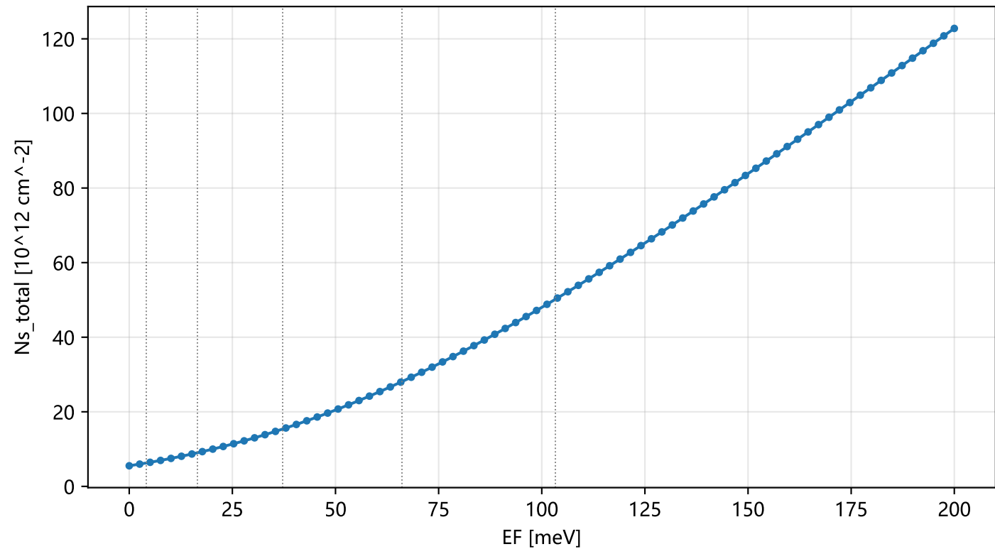
总面密度随费米能级的变化 (虚线为子带能级)
