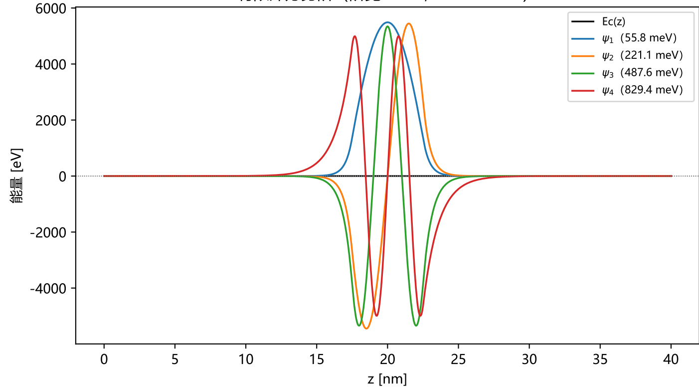
有限深方势阱 (阱宽 5 nm, V_0 = 1.0 eV)
