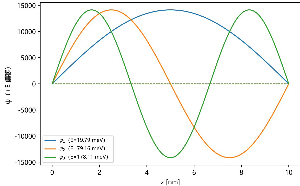
无限深方势阱：波函数 (FDM)
