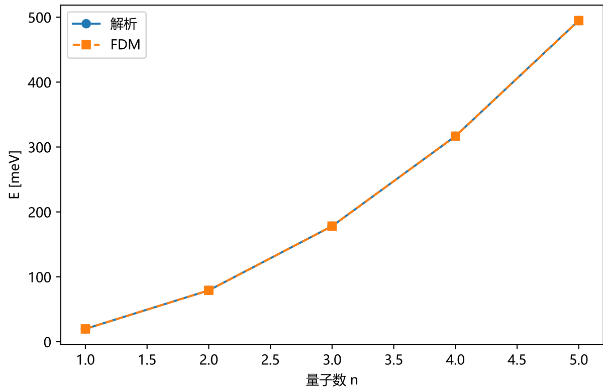
无限深方势阱：能级阶梯
