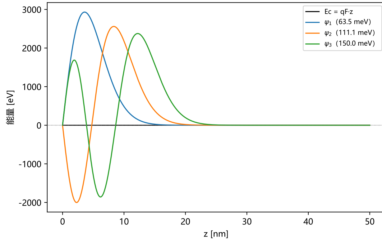
三角势阱：波函数
