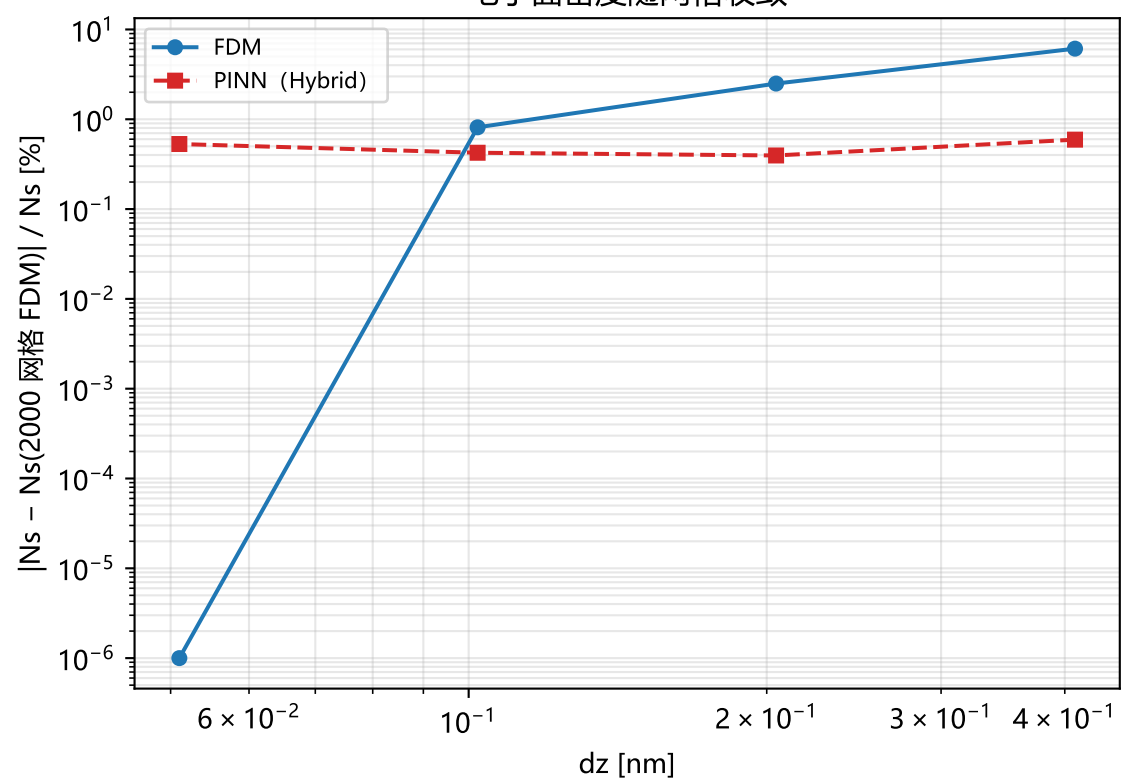
电子面密度随网格收敛
