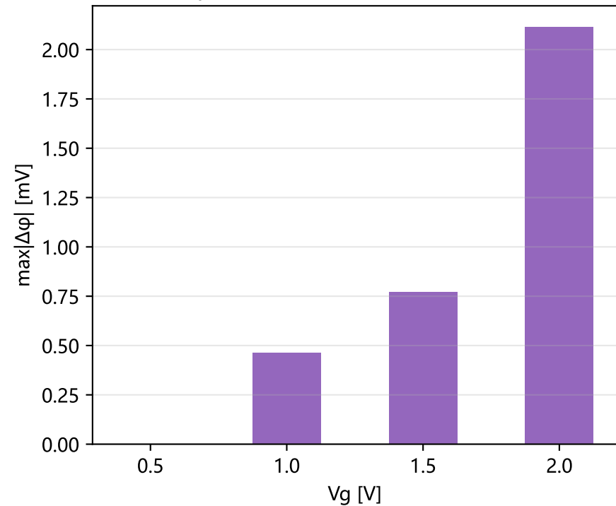
Hybrid 相对 FDM 的逐点最大偏差
