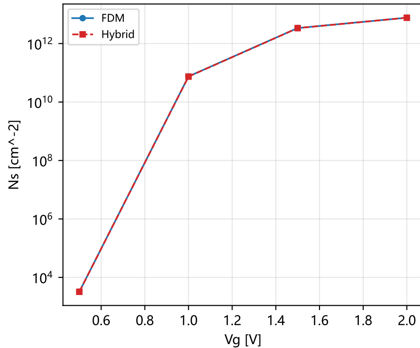
电子面密度对照 (对数)
