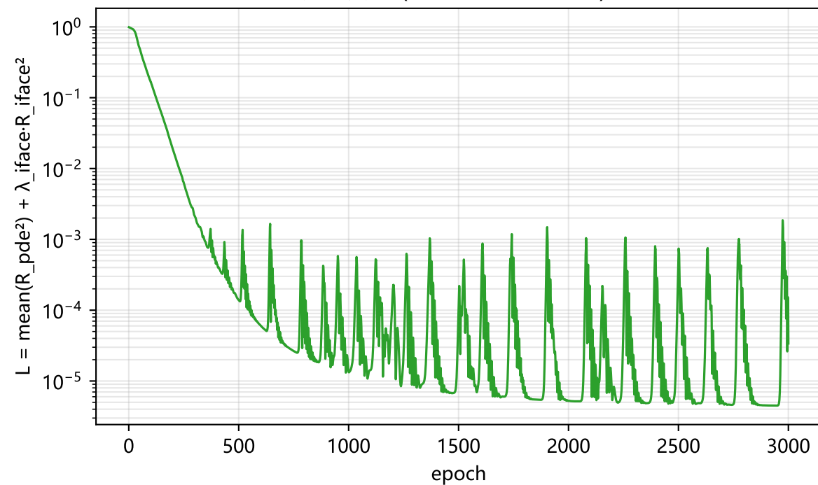
训练损失 (wall time = 40.3 s)
