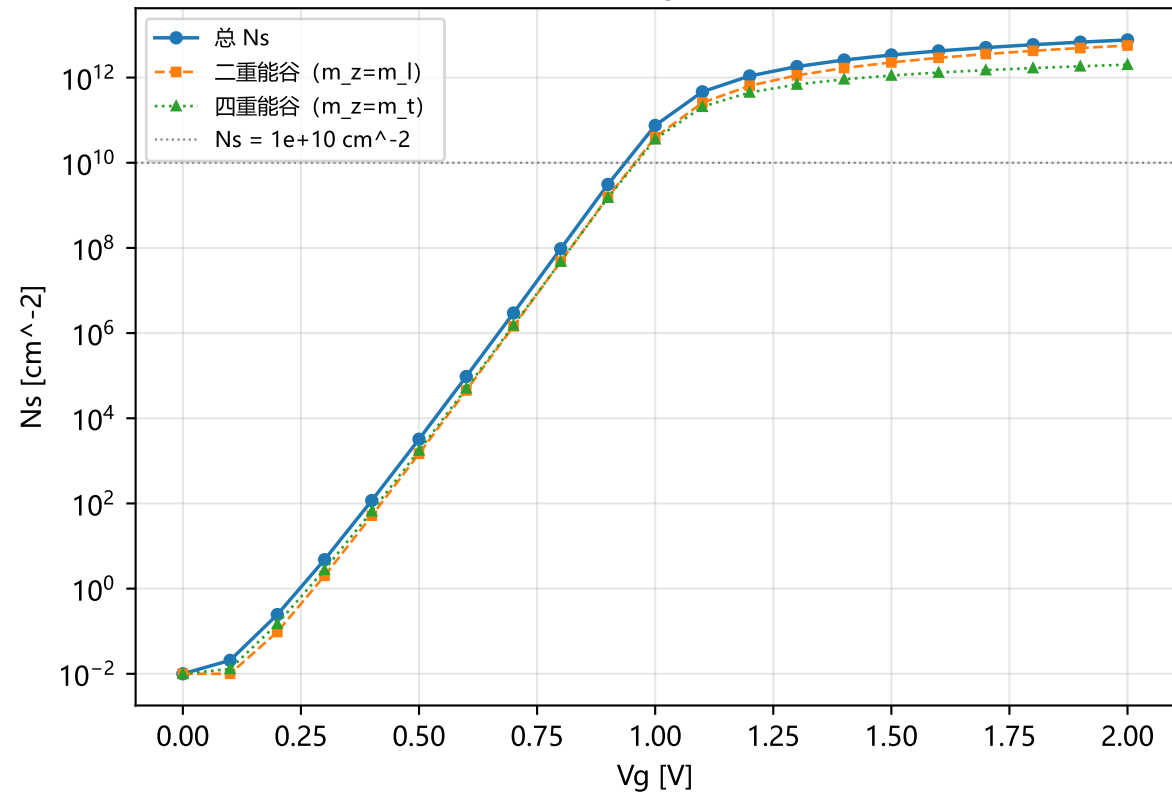
电子面密度随 V_g (对数坐标)
