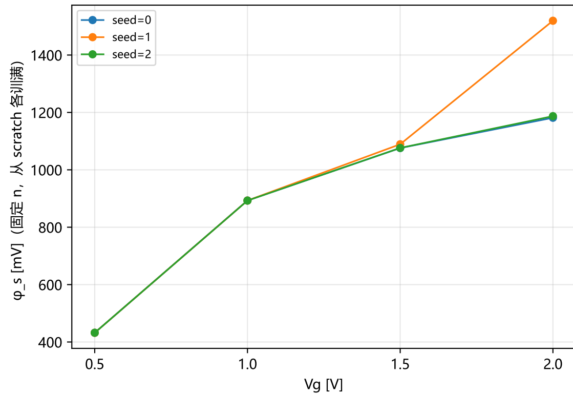
A 组: from-scratch 的 G 漂移 (跨 seed 散布)
