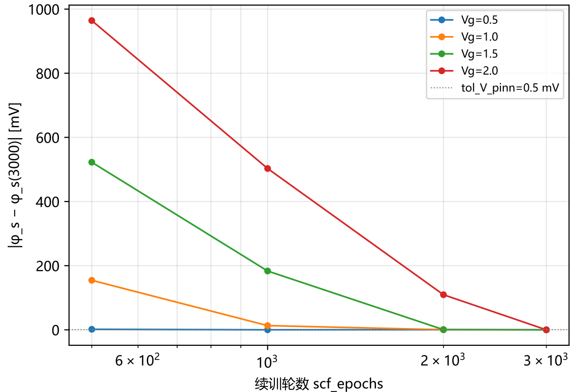
B 组: 轮数不足 \rightarrow G 漂移
