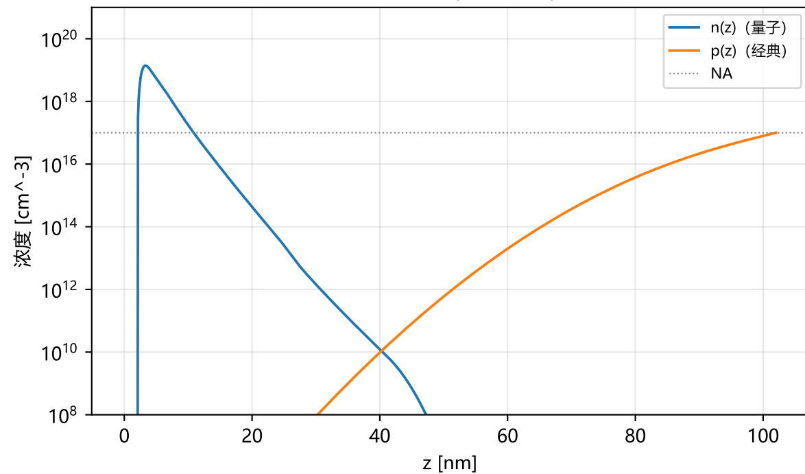
载流子浓度 (对数坐标)
