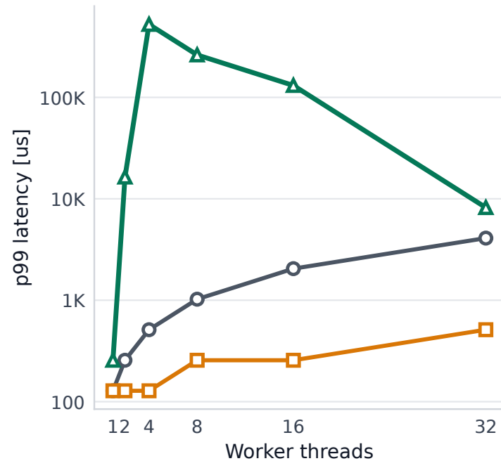
YCSB-A
