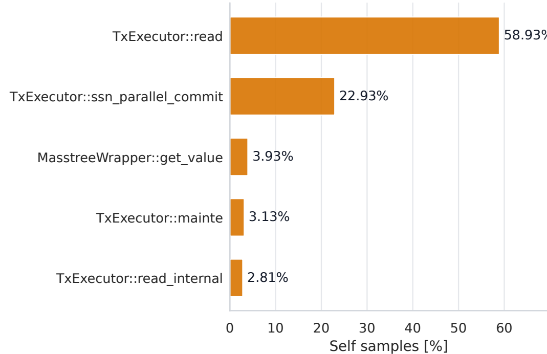
P-WAL
