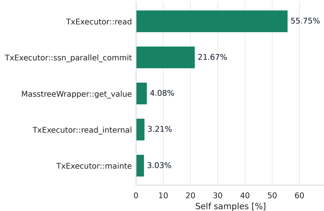
TideWAL
