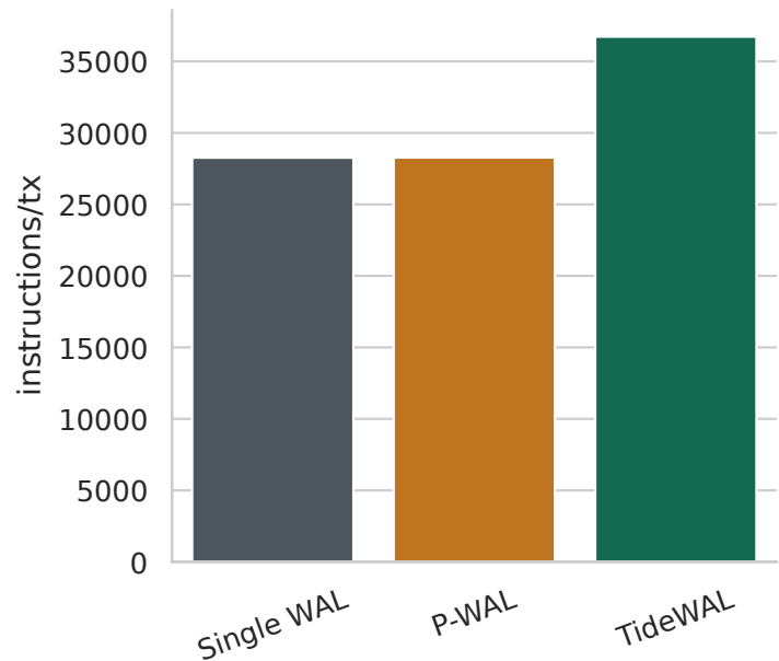
perf instructions
