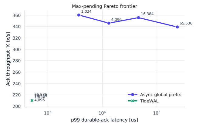
図 6 Max-pending Pareto frontier.
