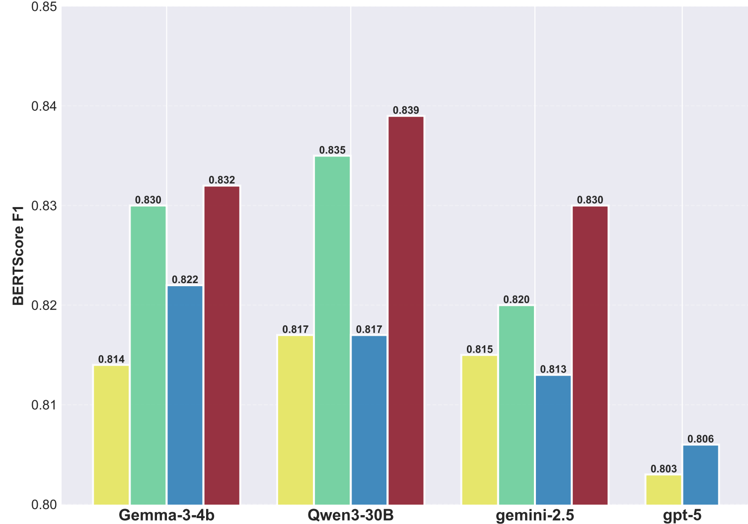
BERTScore F1
