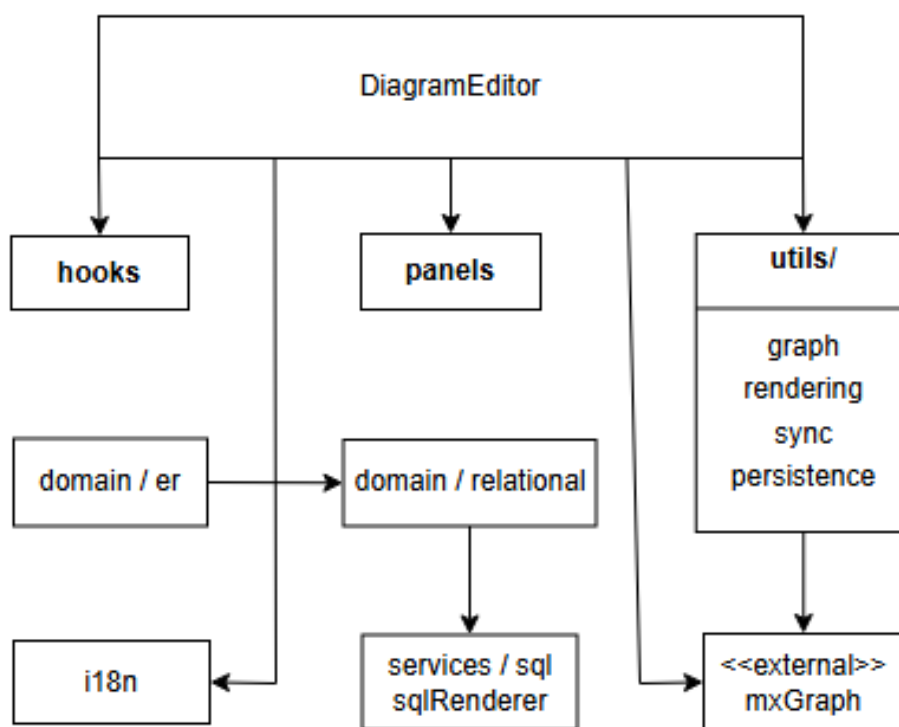
Figura C.5: Diagrama UML de paquetes simplificado de la organización interna de la aplicación.
