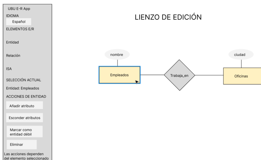
Figura C.9: Boceto de la botonera contextual para una entidad seleccionada.
