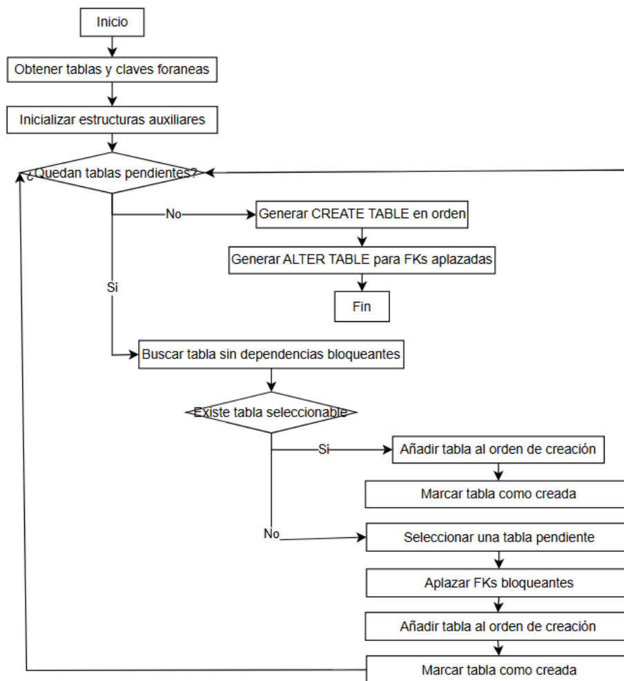
Figura C.6: Diagrama de actividad UML del algoritmo de ordenación de tablas y claves foráneas.
