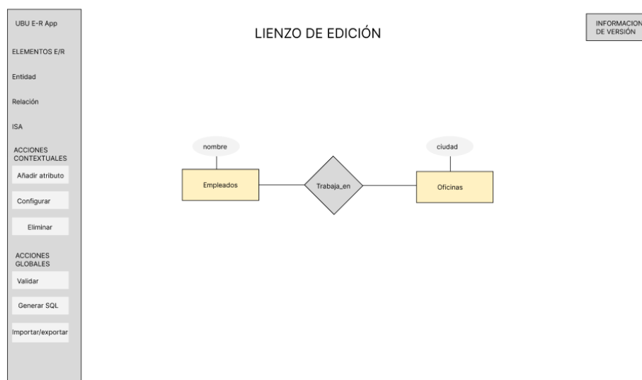
Figura C.7: Boceto de la estructura general de la interfaz del editor.
