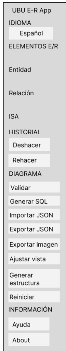
Figura C.8: Boceto de la botonera general del diagrama.
