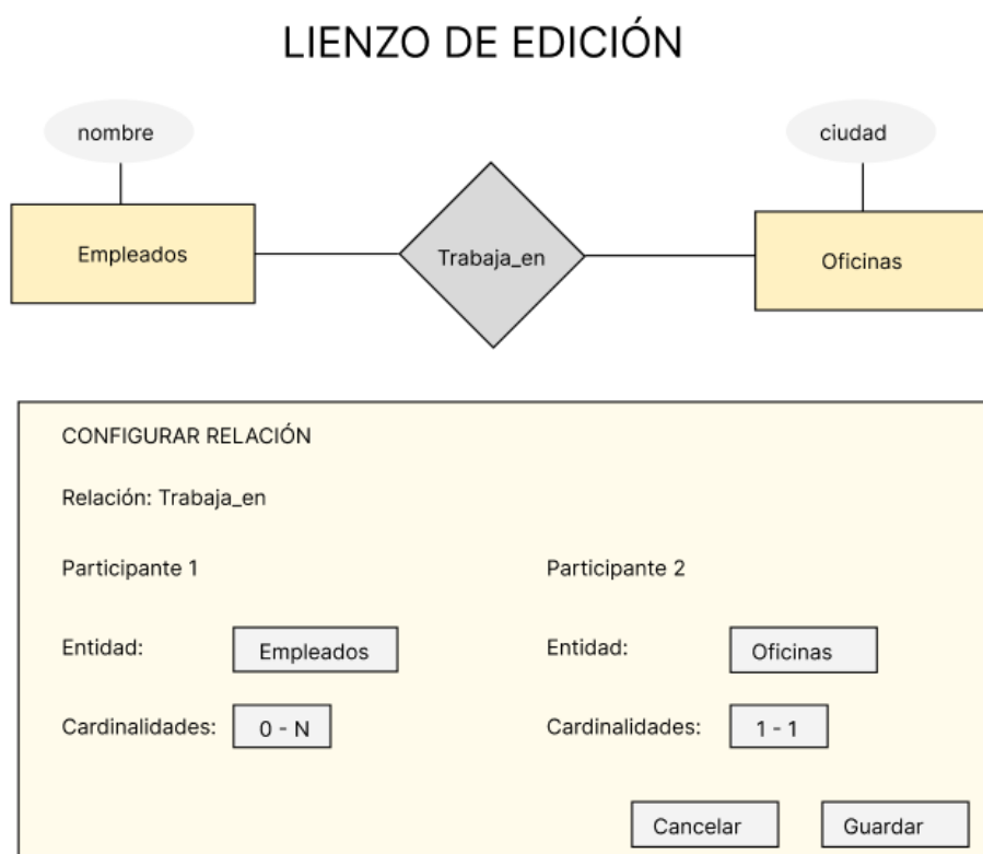
Figura C.10: Boceto de los diálogos de configuración de relaciones y cardinalidades.
