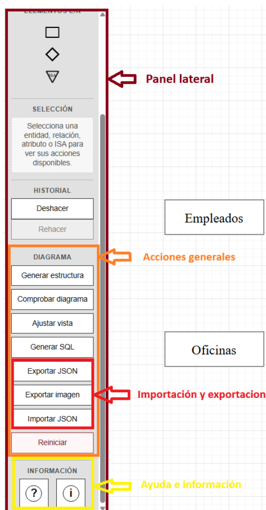
Figura E.3: Panel lateral con acciones generales, importación, exportación y ayuda del editor.
