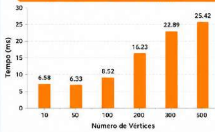
Tempo de Execução – Grafos Densos
