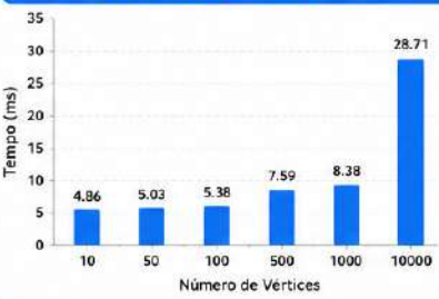
Tempo de Execução – Grafos Esparsos
