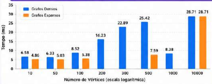
Comparação: Tempo de Execução (ms)
