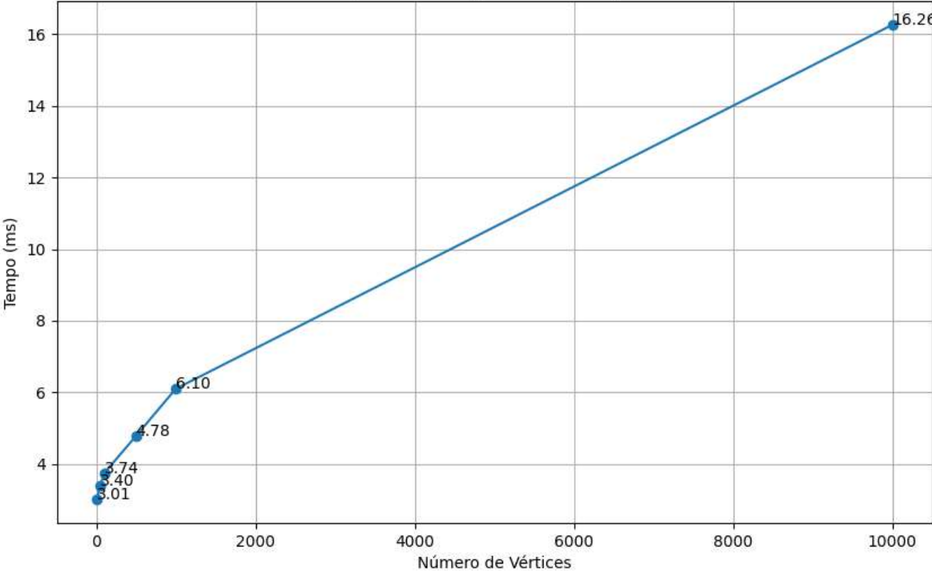
Tempo de Execução - Grafos Esparsos
