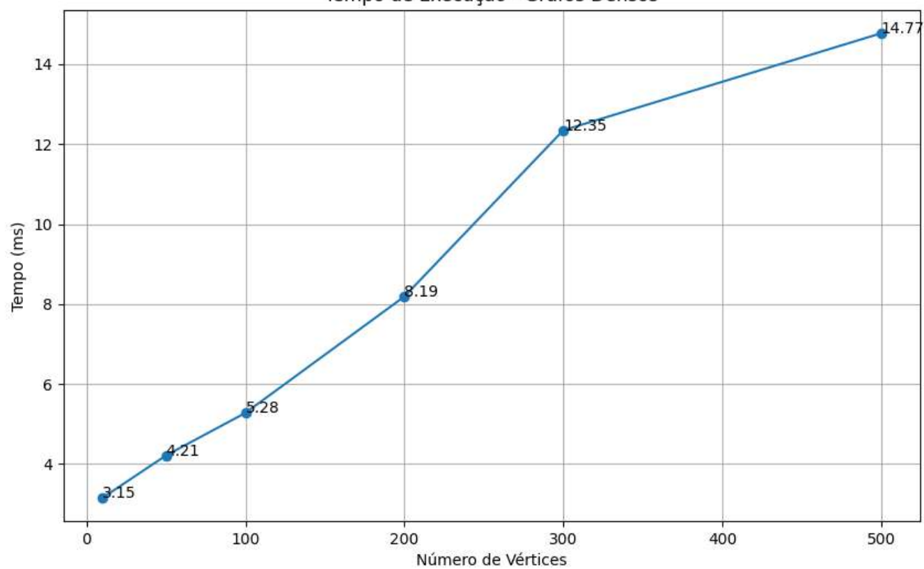
Tempo de Execução - Grafos Densos
