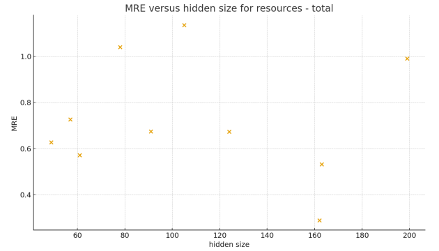
(d) MRE vs Hidden Layer Size: Resources - Total
