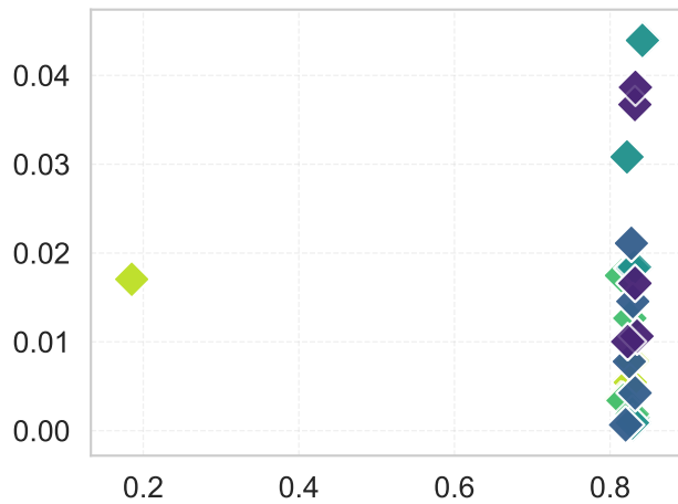
FTL+SDR ξ
