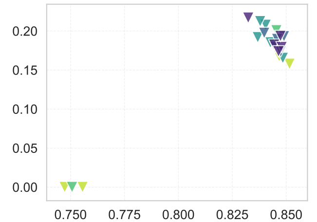
HIFI
