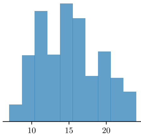
Subset = 0.7
