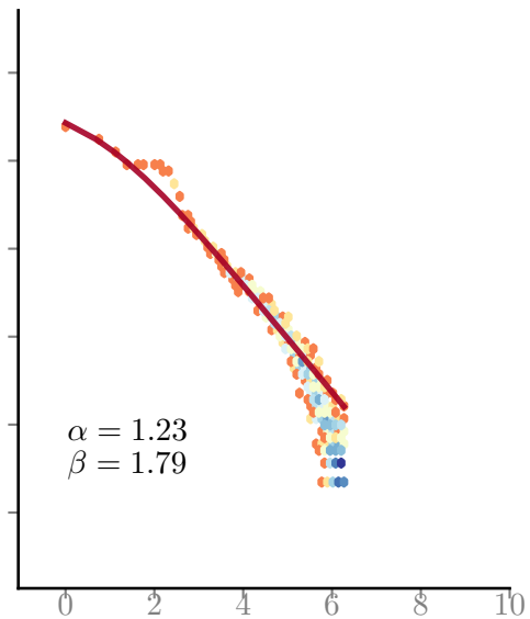
Subset: 0.7
