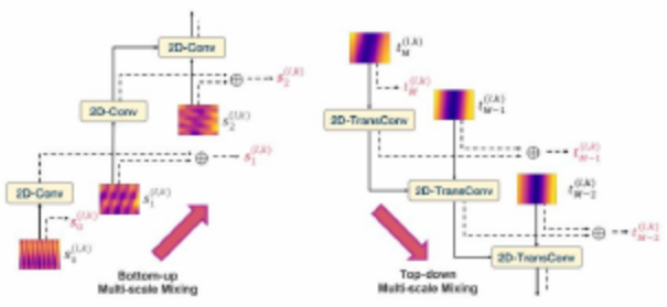
Figure: 多尺度层次混合季节/趋势图像：输出累积先验；自底向上2D卷积，自顶向下反卷积适配尺度。
