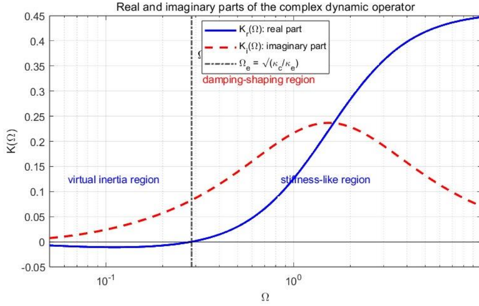
图 3.1 展示了电网络反馈由低频虚拟惯性、过渡区阻尼增强、高频附加刚度三种作用组成，说明复算子不是简单的固定阻尼或固定刚度，而是随频率变化的动力学整形项。
