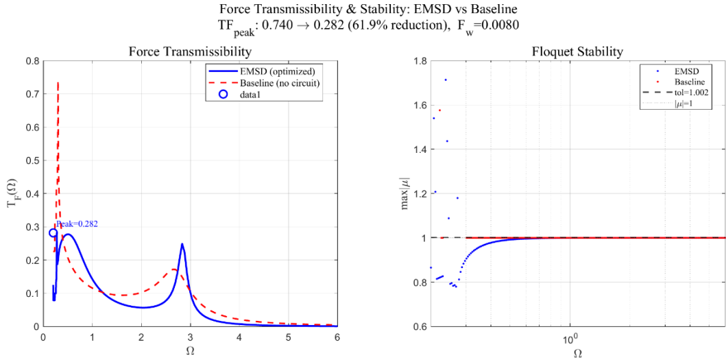
图 3.4 优化参数与纯机械基线的力传递率对比
