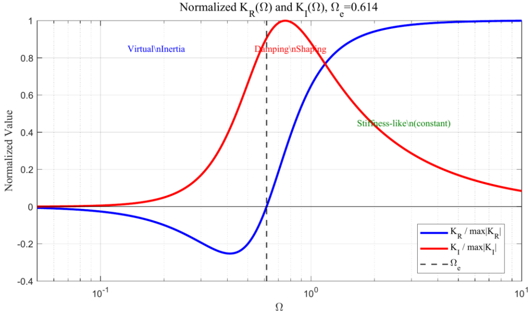
图 3.3 归一化复算子实部与虚部
