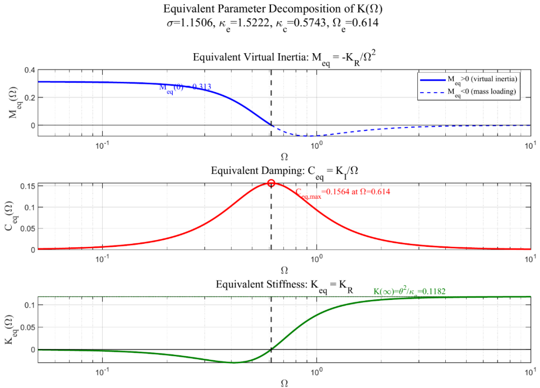
图 3.2 等效惯性 M_{eq} 、等效阻尼 C_{eq} 与等效刚度 K_{eq} 的频率分解
