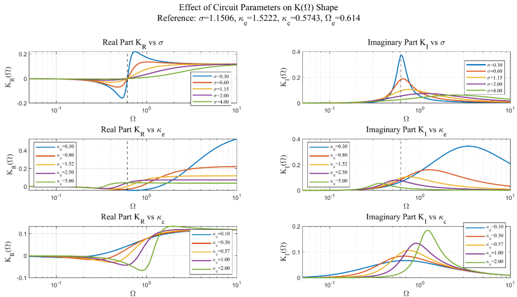
图 3.4 电路参数 \sigma 、 \kappa_e 、 \kappa_c 对复算子实部与虚部的影响
