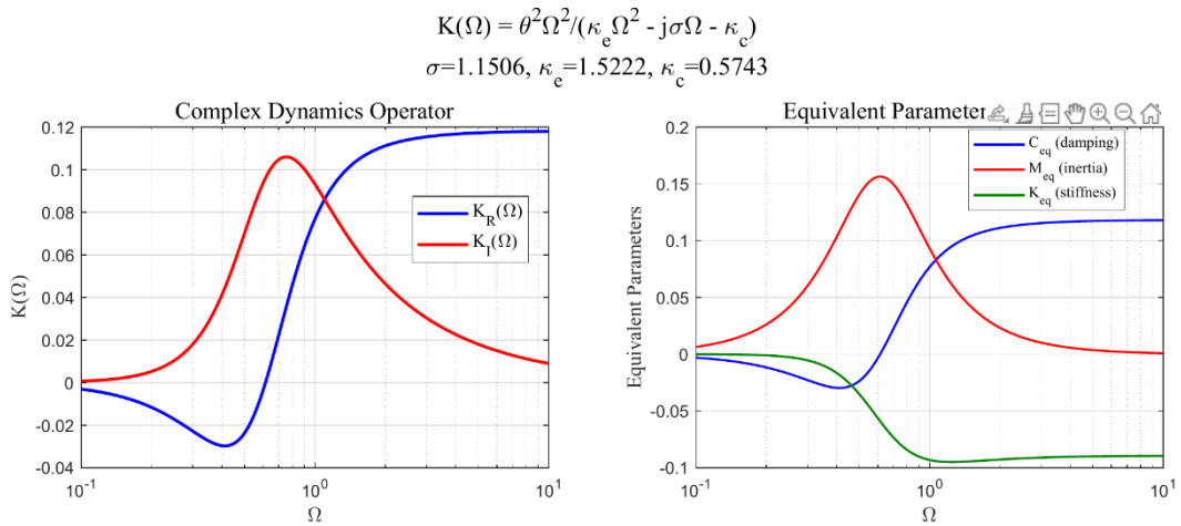
图 3.1 优化参数下的复算子 K(\Omega) 实部与虚部
