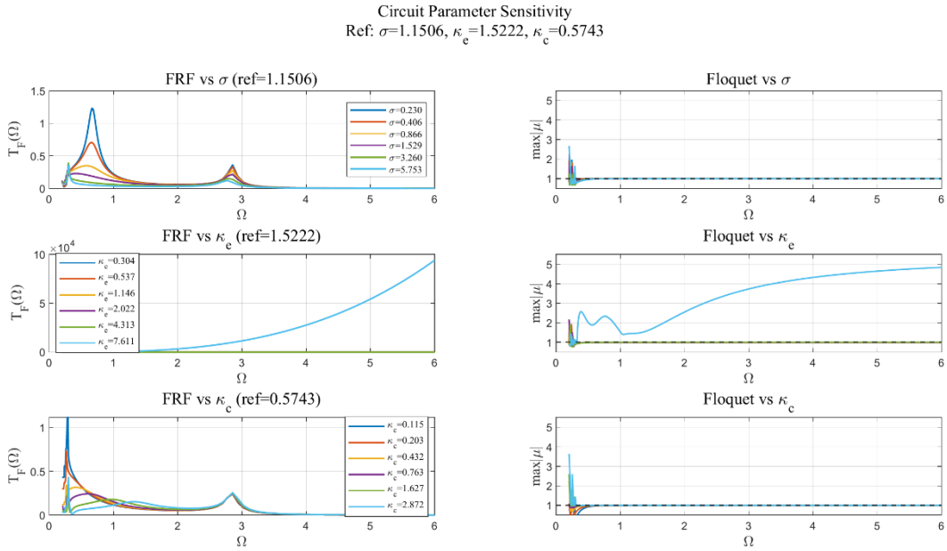
图 3.2 电路参数 \sigma 、 \kappa_e 、 \kappa_c 对幅频响应的扫描结果
