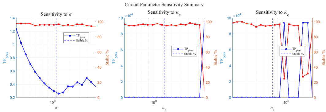
图 3.3 电路参数对力传递率峰值的灵敏度
