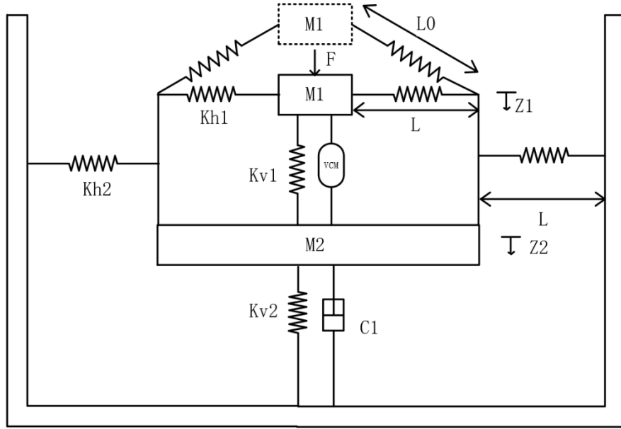
机械结构原理图
