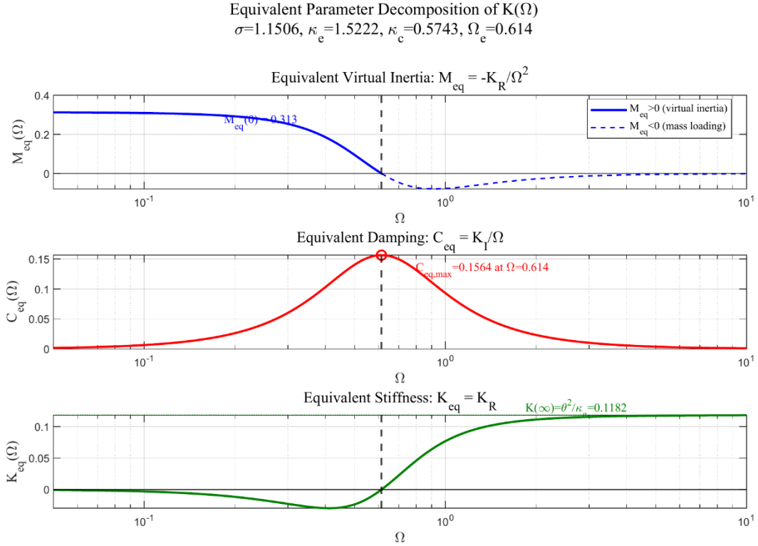
图 4.2 等效惯性 M_{eq} 、等效阻尼 C_{eq} 与等效刚度 K_{eq} 的频率分解
