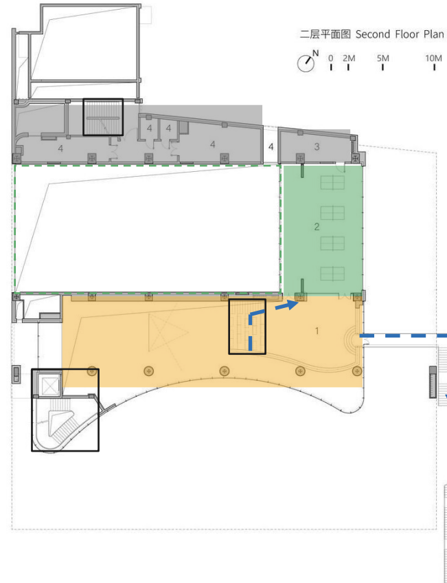
طبقه ۲ - 1 نیم طبقه‌ی فعالیت 2۰ تنیس روی میز 3۰ انبار 4۰ تأسیسات؛ خط چین = فضای تهی استخر در زیر
