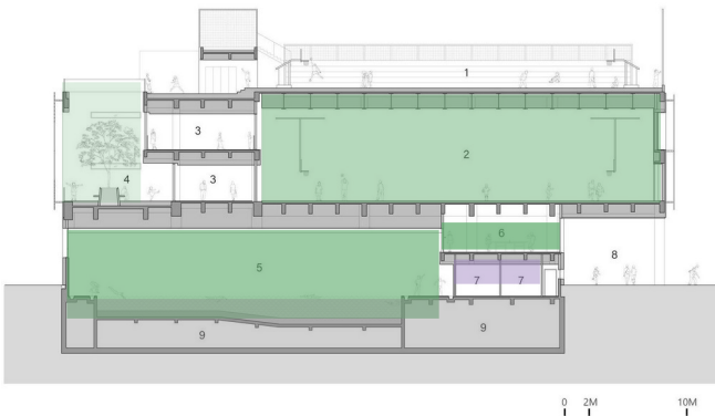
مقطع شمالی-جنوبی (ص. 36) - لایه‌ی تحلیلی از نگارنده
