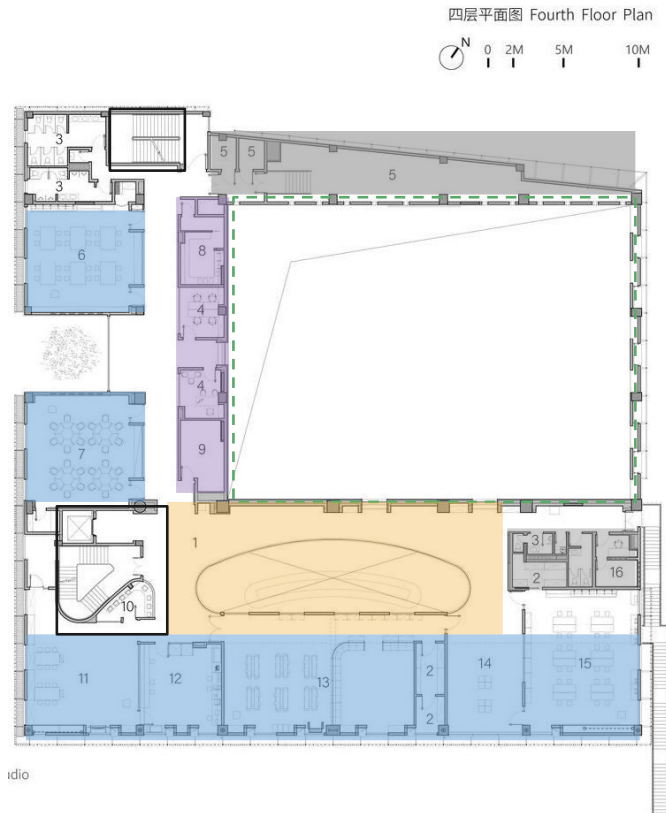
طبقه ۴ - آتلیه‌ها: هنرهای تجسمی، فناوری اطلاعات، ریاضیات، ساخت، چوب، گلخانه، مد، عکاسی، تاریکخانه، چاپ سه بعدی، ضبط صدا؛ خط چین = فضای تهی سالن
