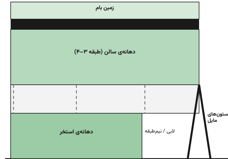
مقطع شماتیک - تفسیر، بدون مقیاس
