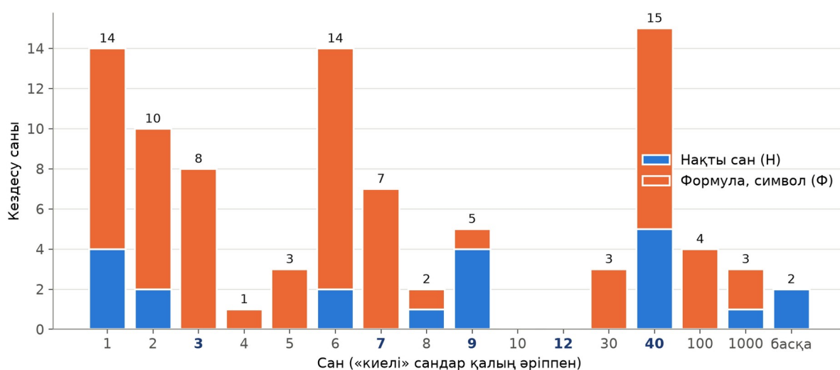
3-сурет – Ертегілердегі сандардың кездесуі
