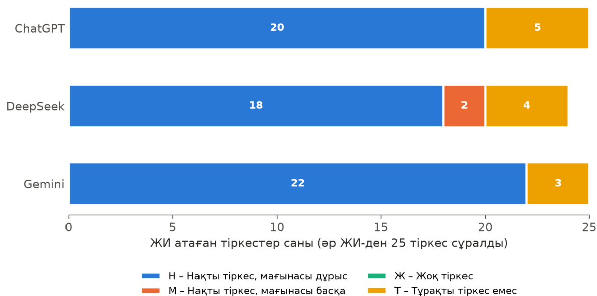
5-сурет – 3-тәжірибе: ЖИ атаған тіркестердің құрамы
